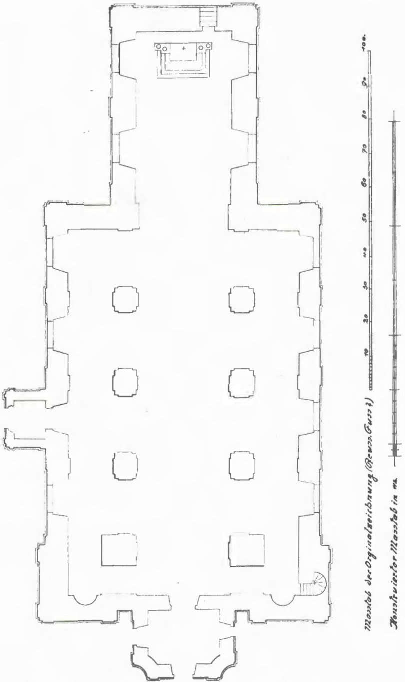
Abb. 2. Grundriß für den geplanten Neubau der Kößeler Jesuitentirche. 18. Jahrh. (1716?). Nicht ausgeführt.
